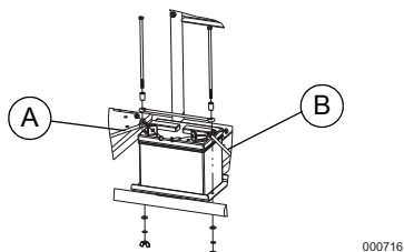
Figura 4-4. Conexión de la batería
