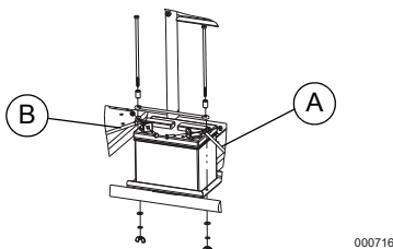
Figura 2-11. Instalación de la batería
